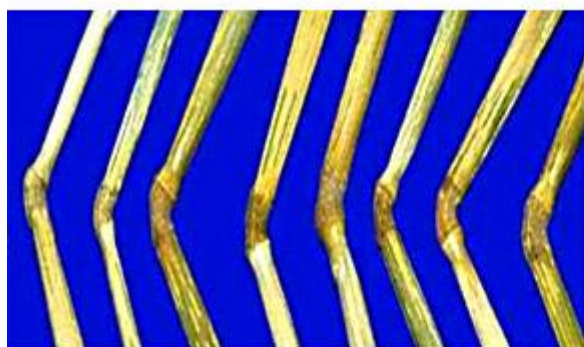
bent nodes
