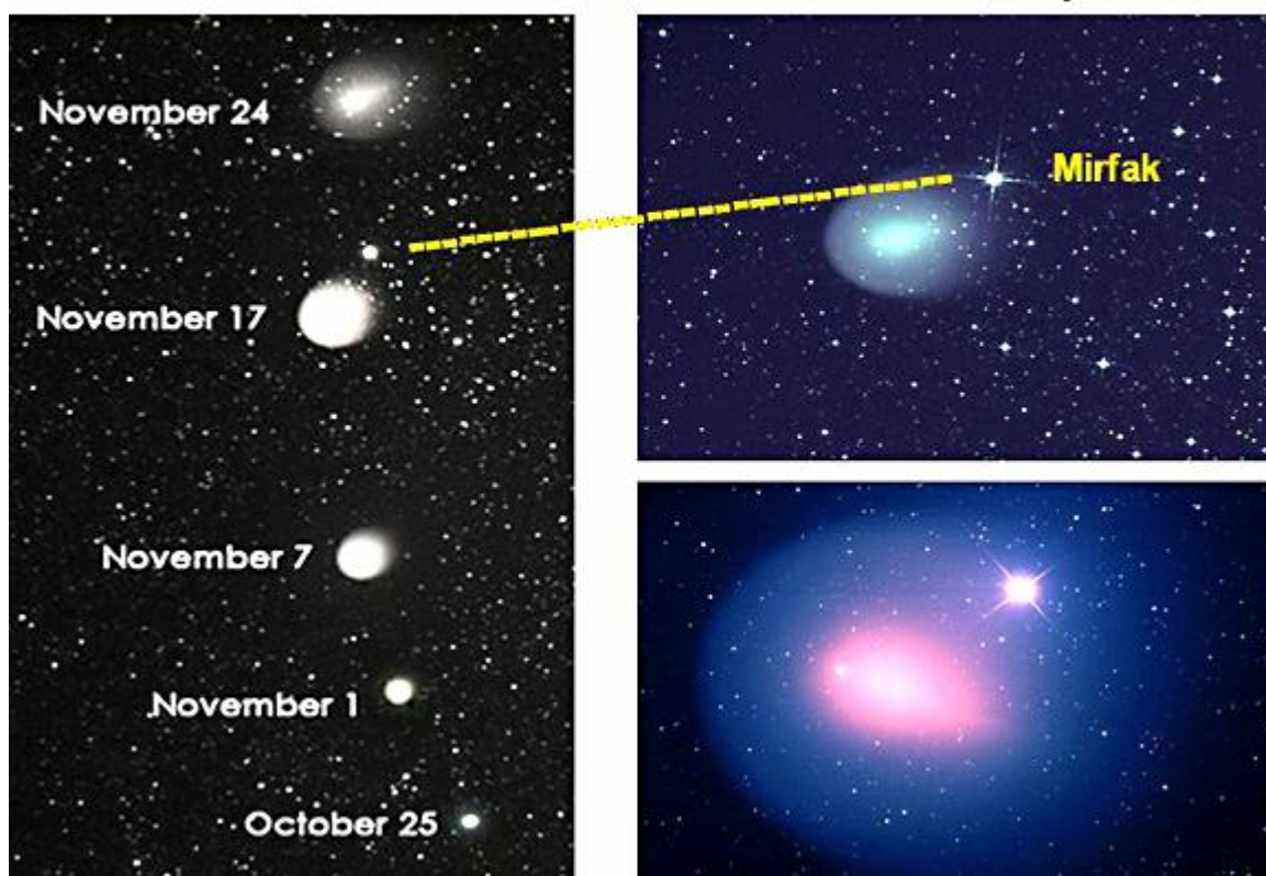
Рис. 48. Соединение кометы Холмса с яркой звездой Мирфак в Персее 20-21 ноября 2007 года.
