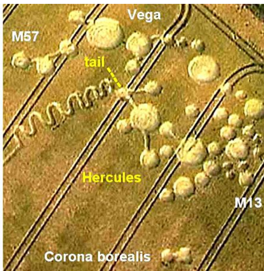
Рис. 40. Звезда в созвездии Геркулеса на расстоянии примерно 160 световых лет от Земли.
