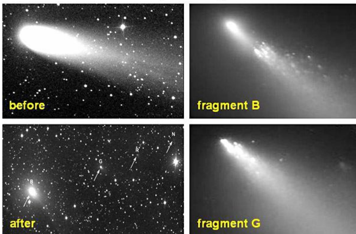
Рис. 45. Три месяца спустя, в сентябре 1995, комета Швассмана-Вахмана 3 взорвалась и рассыпалась на множество маленьких фрагментов вблизи земной орбиты.
